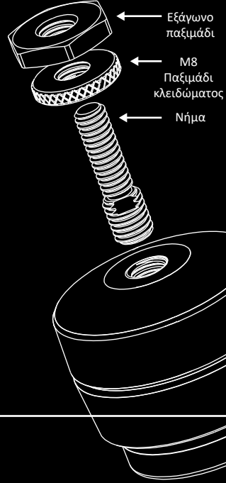
M8 Παξιμάδι κλειδώματος (Qty 4)
