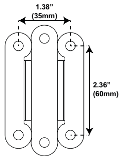
35x60 Adaptador
