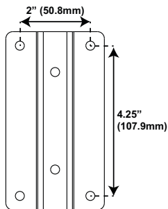
50x107 Adaptador
