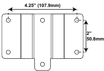
107x50 Adaptador
